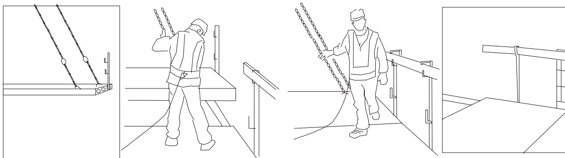
Kuva 18. Elementeissä olevat aukot suojataan välittömästi asennuksen jälkeen suojakaiteilla tai riittävän lujalla kannella. Laatastons asennuksen edetessä reunoille asennetaan kaiteet heti kun mahdollista.
