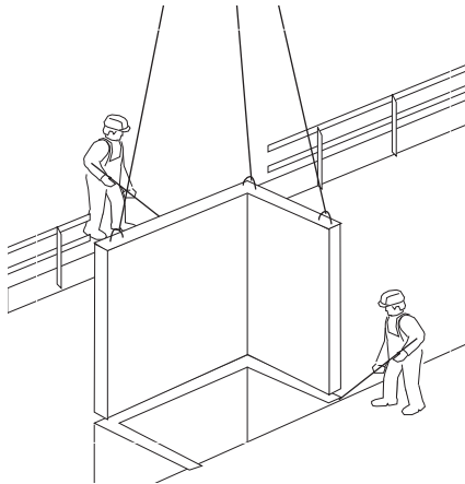
Kuiluelementin asennus.
