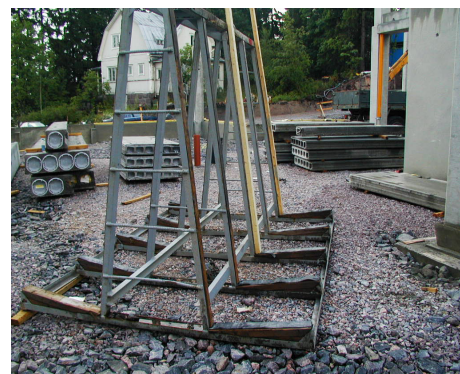
Seinäelementit voidaan varastoida työmaalla esimerkiksi A-pukkeihin. Elementit nostetaan A-pukeista pois vuorotellen kummaltakin puolelta, jotta telineen tasapaino säilyy.
