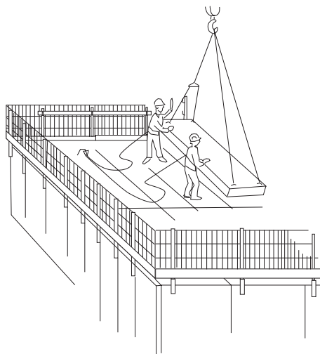
Kaiteet asennetaan työn edetessä.
