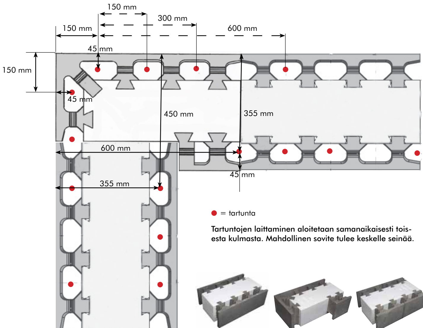
ME400 600 x 400 x 200 mm
